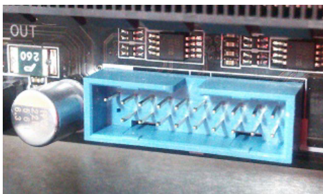
【マザーボードの USB3.0 コネクタ(一例)】
